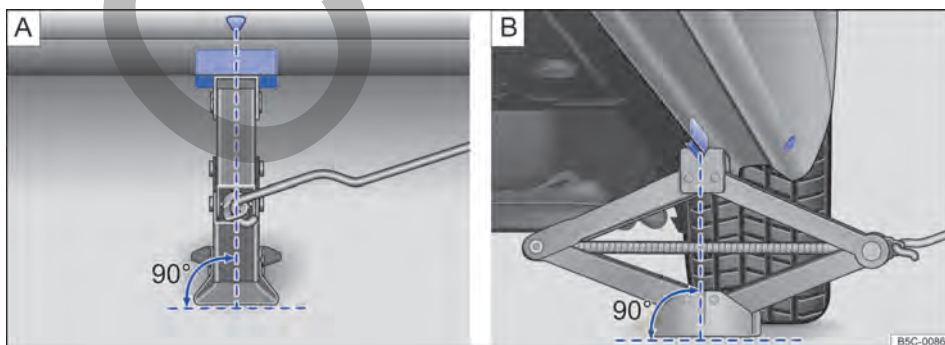
Fig. 205 Gato colocado en el lado izquierdo del vehículo, en la zona trasera.
