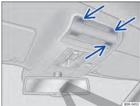
Fig. 65 En la consola del techo: sensores de la vigilancia del habitáculo (flechas).
