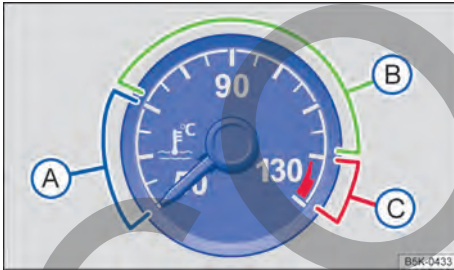
Fig. 15 En el cuadro de instrumentos: indicador de temperatura del líquido refrigerante del motor (representación esquemática).
