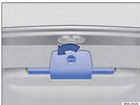
Fig. 53 En el portón del maletero: soporte del triángulo de preseñalización.
