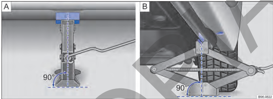
Fig. 207 Gato colocado en el lado izquierdo del vehículo, en la zona trasera.
