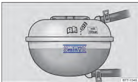
Fig. 186 En el vano motor: marcas en el depósito de expansión del líquido refrigerante del motor (representación esquemática).
