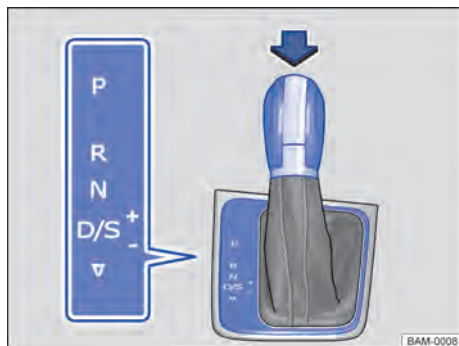
Fig. 108 Vehículo con el volante a la izquierda: palanca selectora del cambio automático con tecla de bloqueo (flecha).
