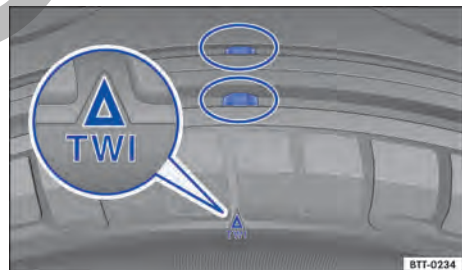
Fig. 195 Perfil del neumático: indicadores de desgaste.
