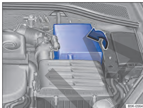
Fig. 190 En el vano motor: abrir la cubierta de la batería de 12 voltios.
