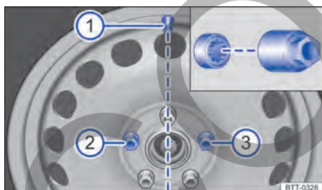
Fig. 203 Cambio de rueda: válvula del neumático ① y lugar de montaje del tornillo de rueda antirrobo ② o ③.
