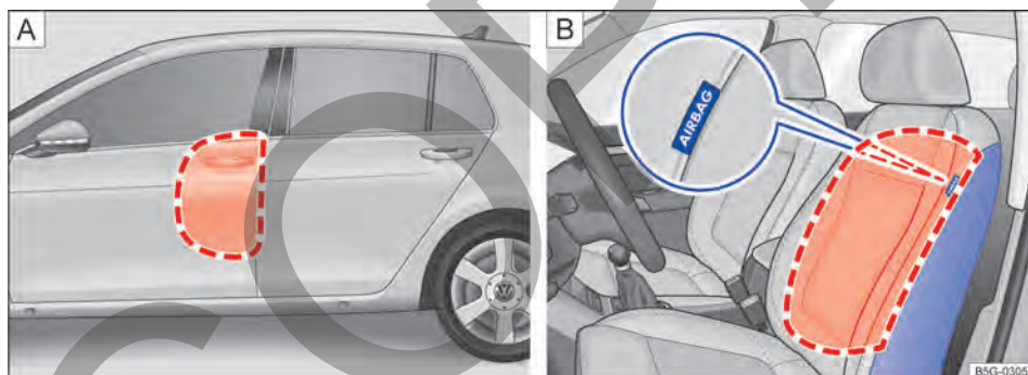
Fig. 42 [A] En el lado izquierdo del vehículo: zonas de despliegue del airbag lateral. [B] Lateral del asiento delantero: ubicación y zona de despliegue del airbag lateral.
