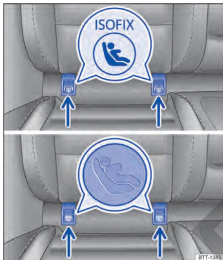
Fig. 49 En el asiento del vehículo: tipos de señalización de los puntos de anclaje ISOFIX para los asientos para niños.
