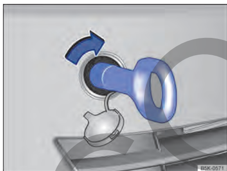
Fig. 179 En el lado derecho del paragolpes delantero: enroscar la argolla de remolque.
