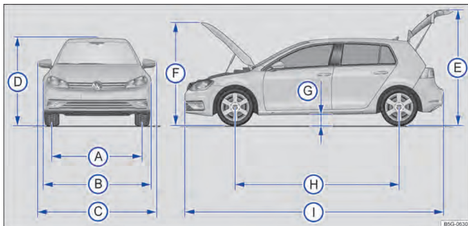
Fig. 216 Dimensiones.
